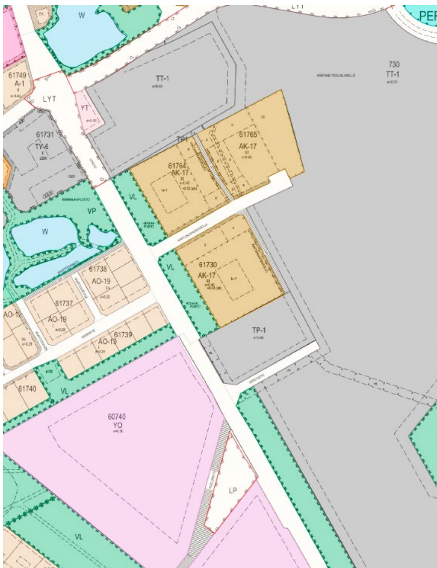
Ote ajantasa-aseamakaavasta (20.6.2023)
